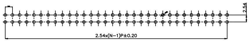
P.C.B LAYOUT
